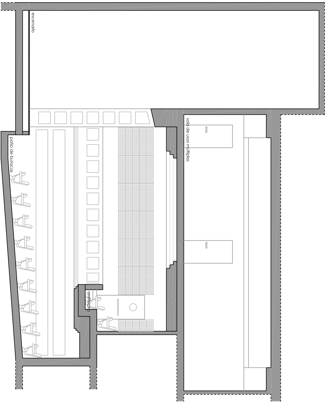
sección cc'
